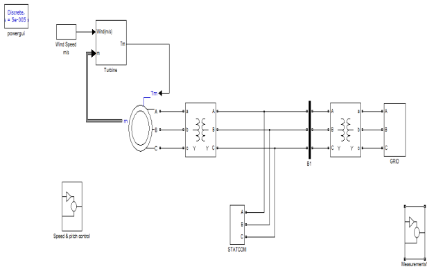
Fig. 9 SCIG Simulink Circuit
