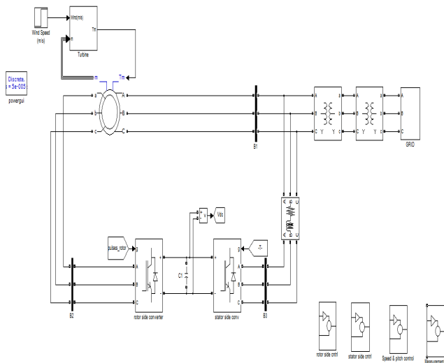
Fig. 11 DFIG Simulink Circuit
